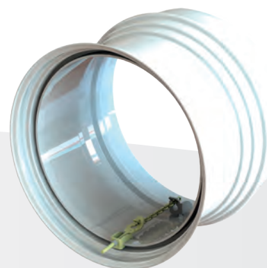
Välivanteen kiinnitys ketjulla. Helpottaa parinpyörän asennusta välivanteen pysyessä paikallaan.
